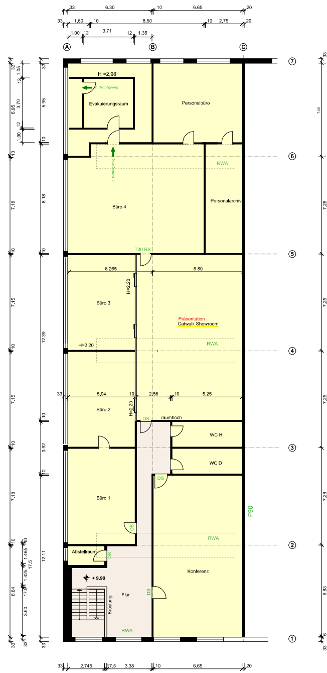
GRUNDRISS 2. Obergeschoss
