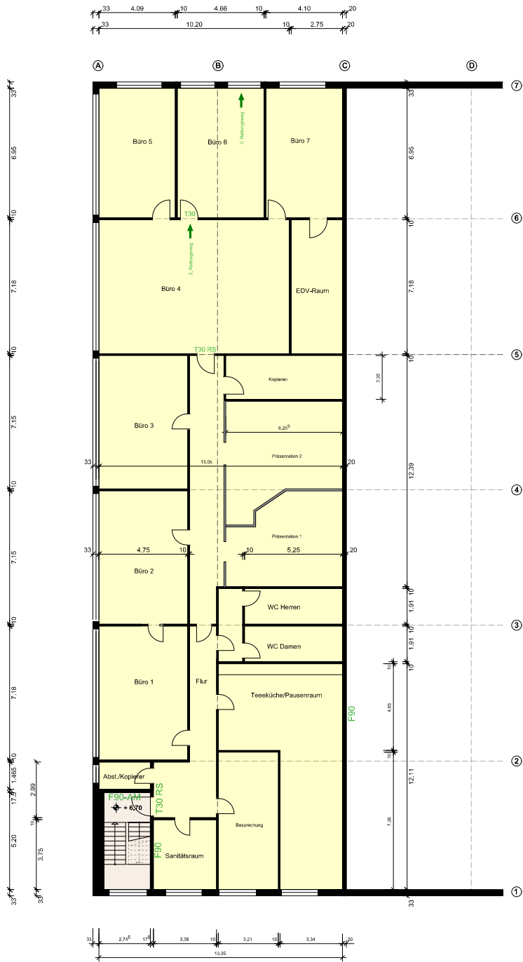
GRUNDRISS 1. Obergeschoss
